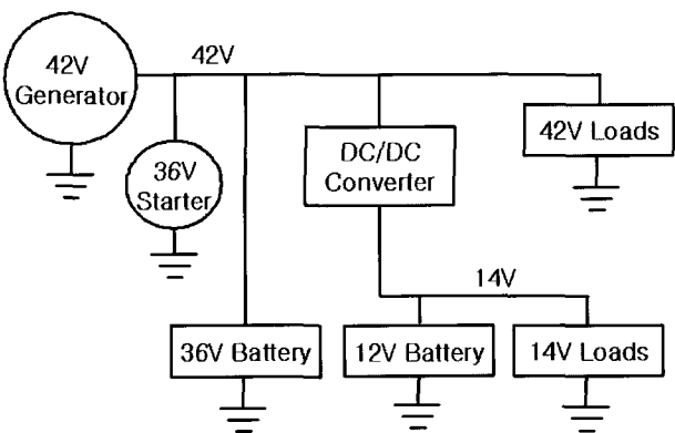
그림 4 DC/DC Converter 이중전압 구조
