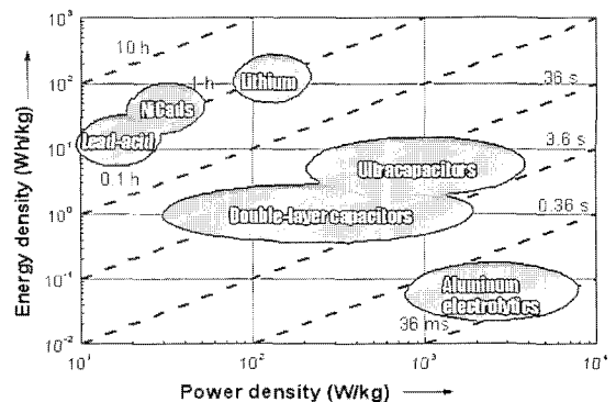
그림 5 에너지 저장 장치의 출력 특성
