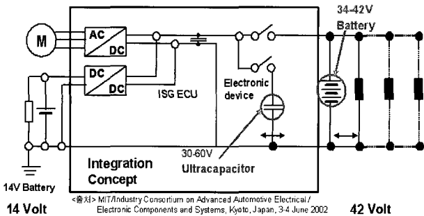
그림 6 42V 전원체계 구성 예
