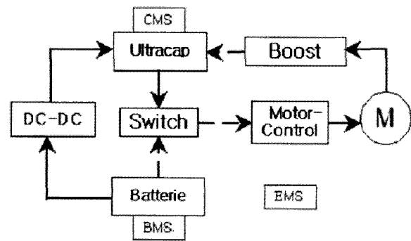
그림 7 DC/DC 컨버터와 Switch를 이용한 저장장치
