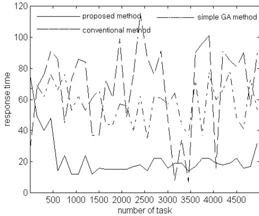
<그림 6> 실험 1에 대한 결과
