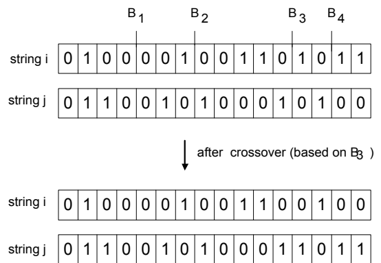
<그림 4> 교배 연산
