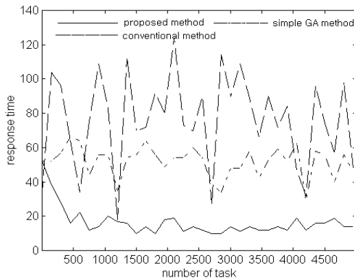
<그림 9> 20%일 때 반응 시간
