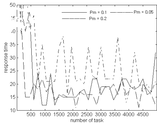
<그림 8> P_m 변화에 따른 실험 결과
