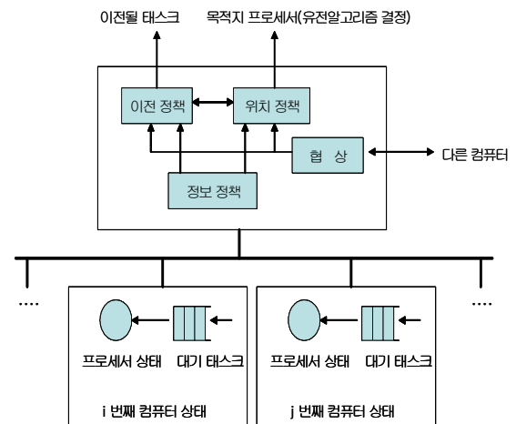
<그림 2> 부하재분배 구성요소
