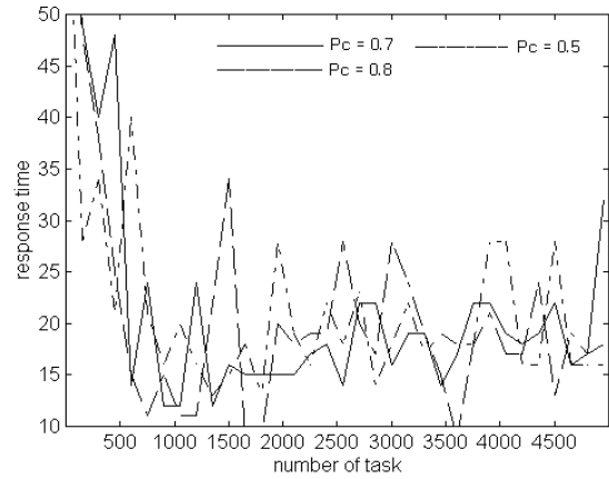
<그림 7> P_c 변화에 따른 실험 결과
