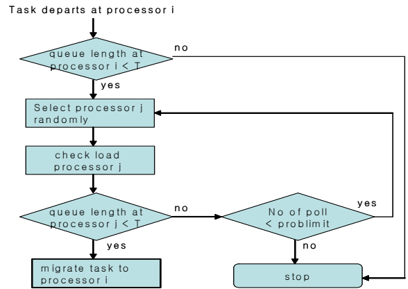
<그림 1> 수신자개시 부하재분배 알고리즘
