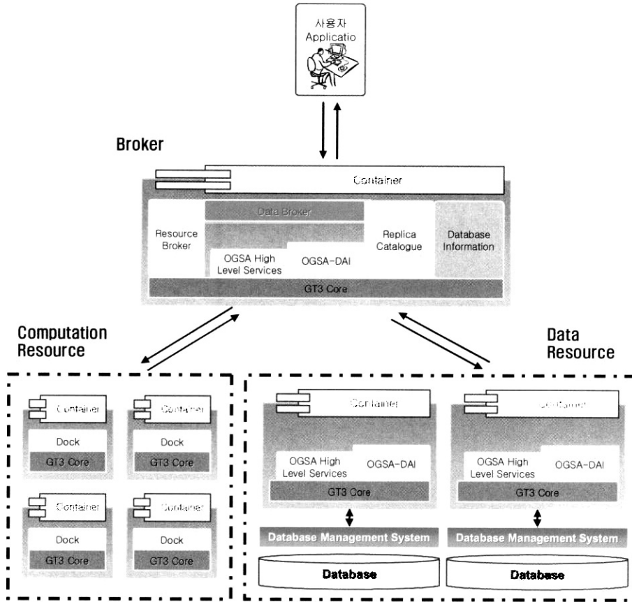
<그림 2> 서비스 기반 분자 모델링 시스템의 전체 구조
