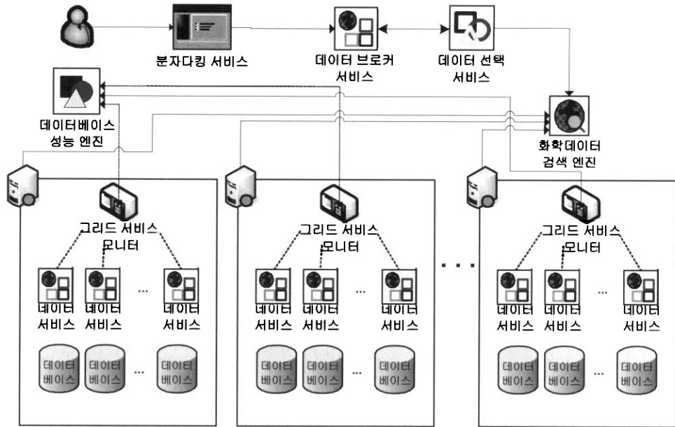
<그림 4> 데이터 브로커의 구성 요소
