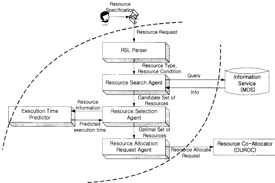
<그림 3> 최적 자원 선택 브로커의 구조
