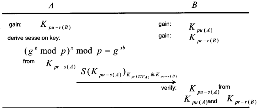
그림 1. RHP 프로토콜
