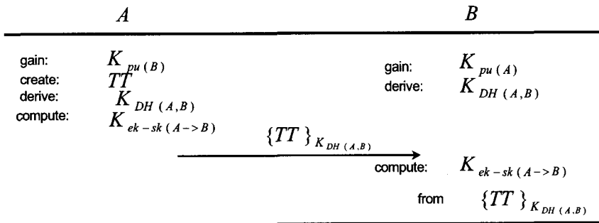
그림 3. 제안한 프로토콜
