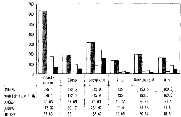
(그림 5) 메모리 사용량
