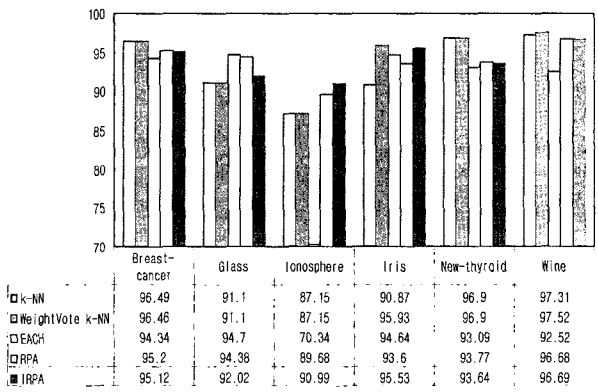
(그림 4) 분류 성능
