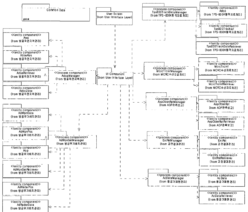
(그림 3) 항적추적관리시스템 컴포넌트 구조
