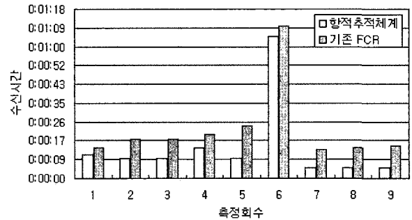
(그림 8) 레이더자료의 실시간 상황도도시와 FCR 수신시간 비교
