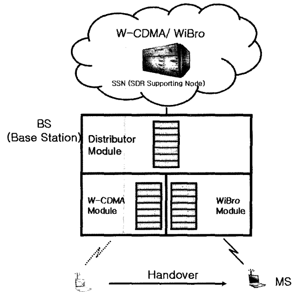
(그림 1) 전체 시스템 구조
