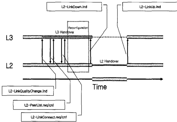
(그림 1) L2, L3 및 제한한 핸드오버 프로토콜의 관계
