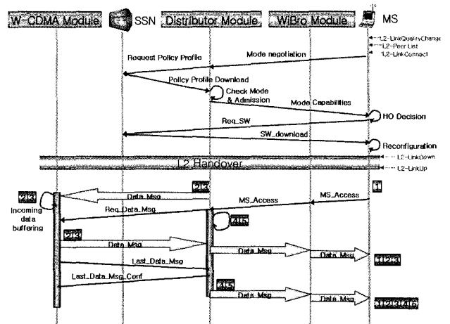
(그림 2) 이중모드를 지원하는 기지국 내에서의 핸드오버 프로토콜 절차
