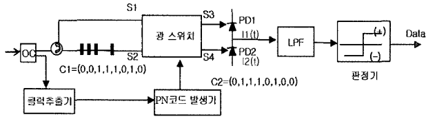
(그림 3) OCD 의 구성
