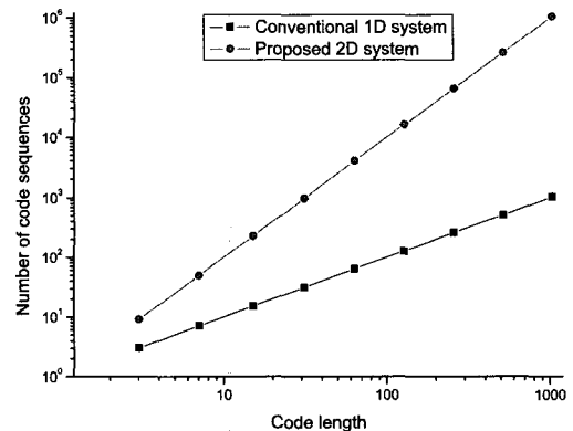
(그림 4) 수정한 PN 코드의 부호장에 대한 생성 가능한 부호의 수
