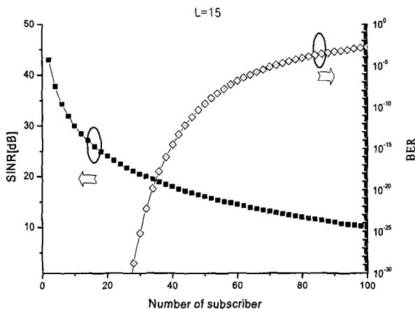
(그림 6) 가입자 수에 따른 SINR 및 BER 특성
