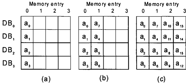
(그림 1) 16-point FFT를 위한 첫 번째 스테이지에서 DB를 위한 Data permutation (클럭 사이클 (a) t=i , (b) t=i+1 , (c) t=i+3 )
