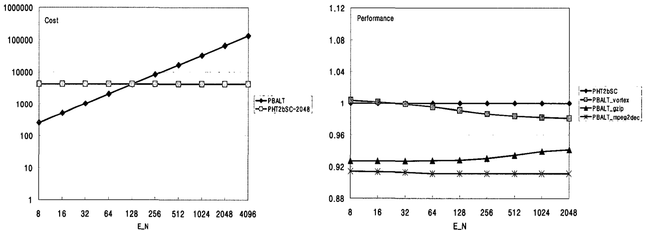
(그림 13) h/w 비용과 성능 비교
