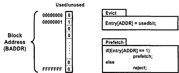
(그림 5) 완전 블록 주소 테이블 구조(CBAT)
