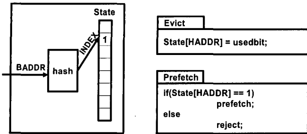
(그림 4) 선인출 해싱 테이블 1bitSC 구조(PHT1bSC)
