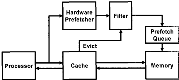
(그림 2) 필터링을 적용하는 하드웨어 선인출 구조
