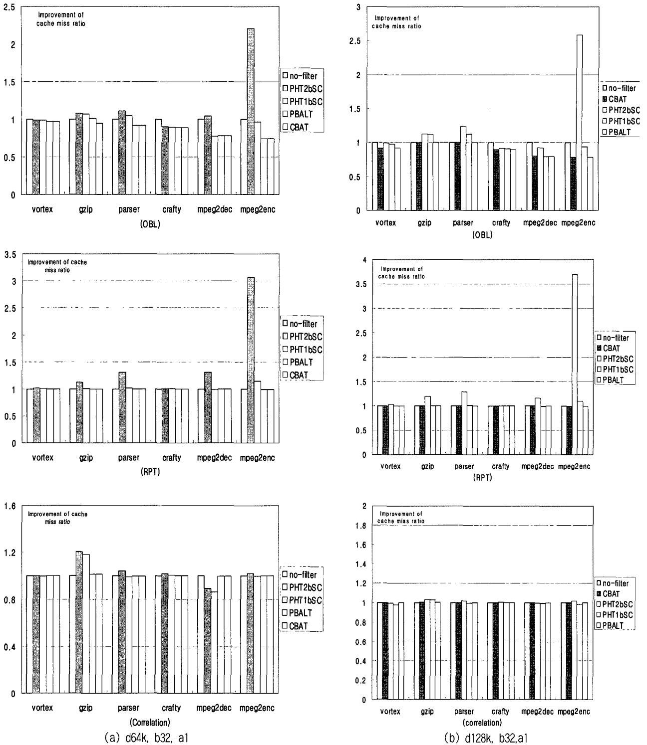
(그림 11) 벤치마크별 캐시 미스 수
