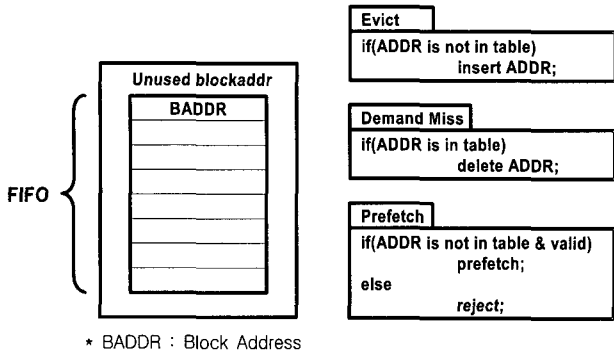
(그림 6) 선인출 블록 주소 참조 테이블 구조(PBALT)
