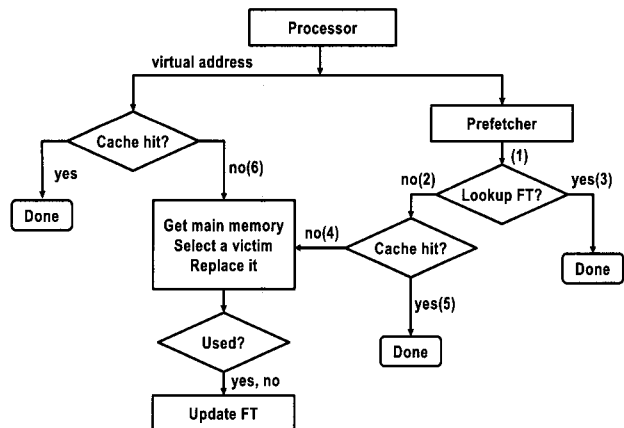
(그림 8) 선인출 명령 발생을 위한 필터 구조를 포함한 흐름도
