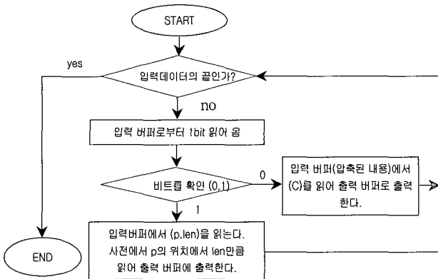
(그림 2) 압축 파일 시스템에서 압축 해제 과정
