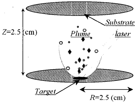
그림 1. 방전 챔버 모델. 방전 챔버의 높이 Z=2.5 cm, 챔버의 반경 R=2.5 cm, 가스압력 P=\text{Vacuum} ( 10^{-5} Pa)~66 Pa.
