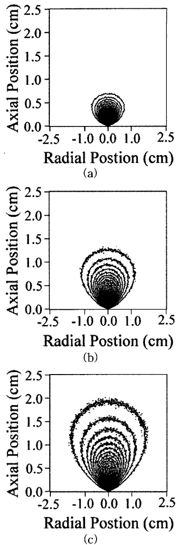
그림 5. Ar 기체압력 P=1 Pa 조건하에서의 탄소 입자의 진전 과정. (a) 100 ns, (b) 500 ns, (c) 100 \mu s. 각각의 등고선은 최대값(6,250)과 최소값(125)을 50등분한 것. Fig. 5. The progress of carbon particles at (a) 100 ns, (b) 500 ns, and (c) 100 \mu s at P=1 Pa of Ar gas. The increment of the contour is 1/50 of the maximum value (6,250).
