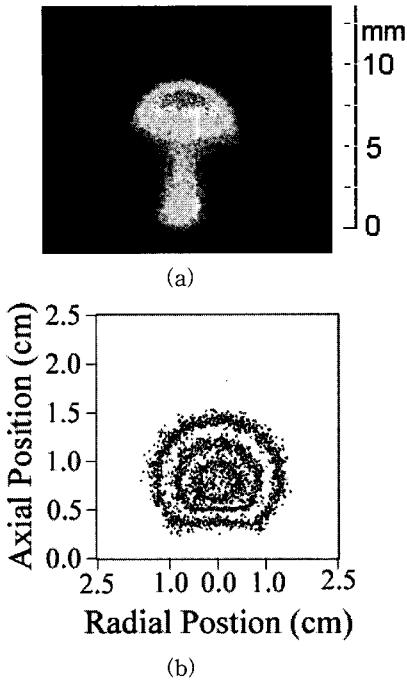
그림 4. 질소 기체 P=10 Pa 압력하에서 530 ns 경과시의 레이저에 의해 발생된 플라즈마 형상. (a) C_2 와 CN 입자의 발광 CCD 화상, (b) 탄소원자의 시뮬레이션 결과. Fig. 4. The ablation plasma distributions of (a) CCD picture of C_2 and CN particles and (b) C atoms over 2.4 eV energy in N_2 gas at P=10 Pa and t=530 ns.
