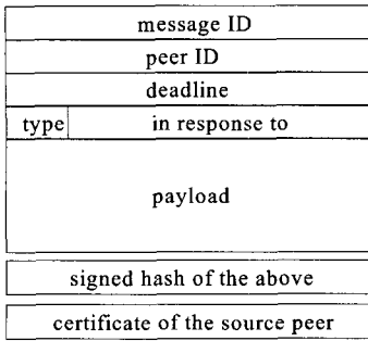
그림 2. 메시지 구조
