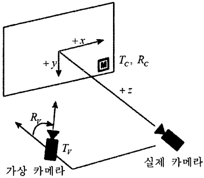
그림 5. 가상 카메라로의 변환
