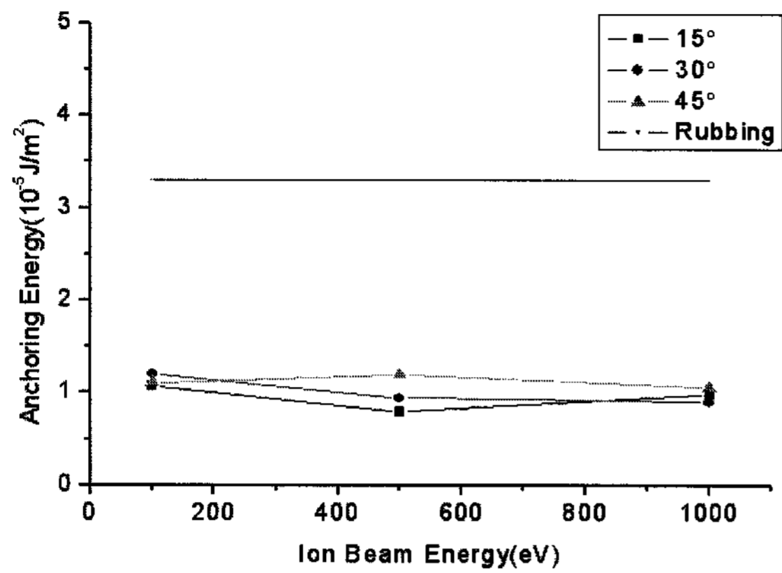
(d) Azimuthal anchoring energy for PIA-5310
