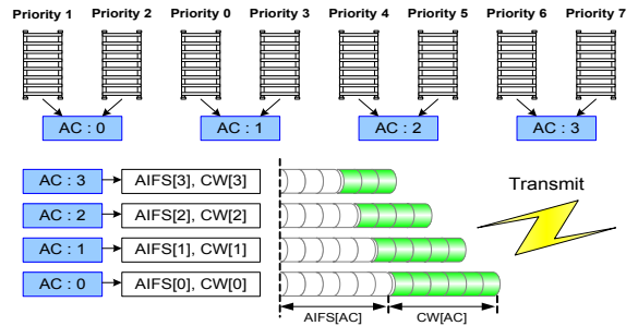
그림 3. IEEE 802.11e EDCF의 동작 과정 Fig. 3. Operation of IEEE 802.11e EDCF mechanism.
