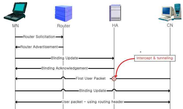
그림 1. Mobile IP 메시지 흐름 Fig. 1. Mobile IP message flow.
