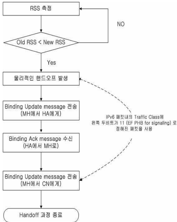
그림 5. 제안하는 알고리즘 Fig. 5. Proposed Algorithm.
