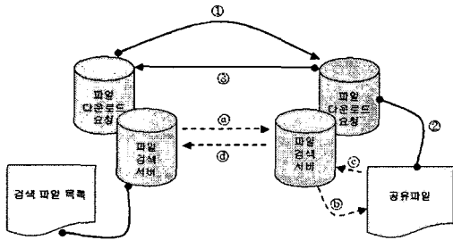
(그림 4) 파일검색과 다운로드
