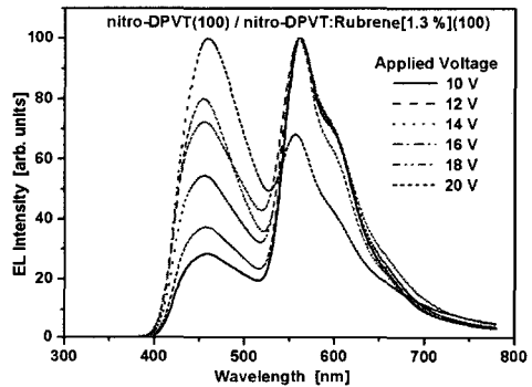
그림 5. 인가전압 변화에 따른 정규화된 EL 스펙트럼(Rubrene의 도핑농도 : 1.3 %).
