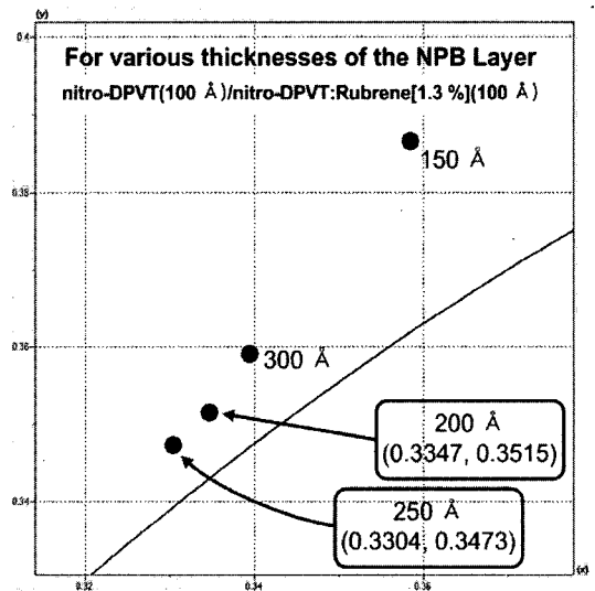
그림 7. NPB층 두께 변화에 따른 CIE 색좌표. Fig. 7. CIE coordinates of devices for various thicknesses of the NPB layer.
