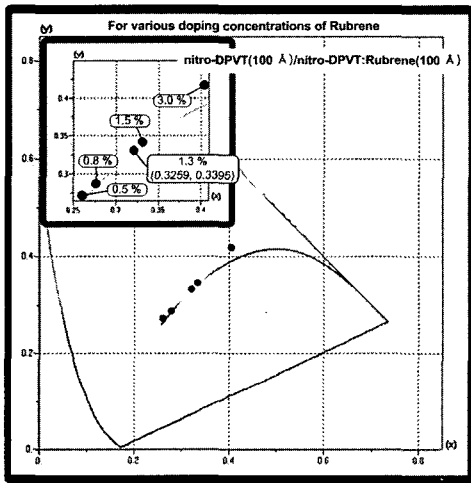
그림 4. Rubrene의 도핑농도 변화에 따른 CIE 색좌표.
