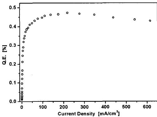
그림 9. 외부양자효율 특성. Fig. 9. External quantum efficiency characteristics of the fabricated white OLED.
