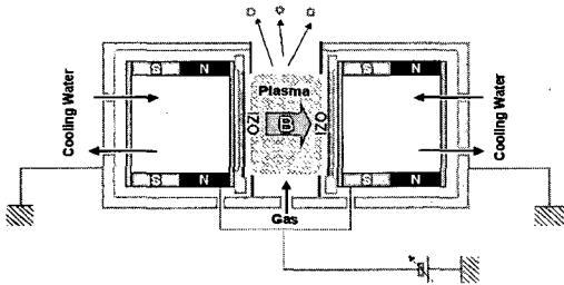
그림 1. OLED용 박스 캐소드 건의 개략도. Fig. 1. Schematics of a box cathode gun for OLEDs.
