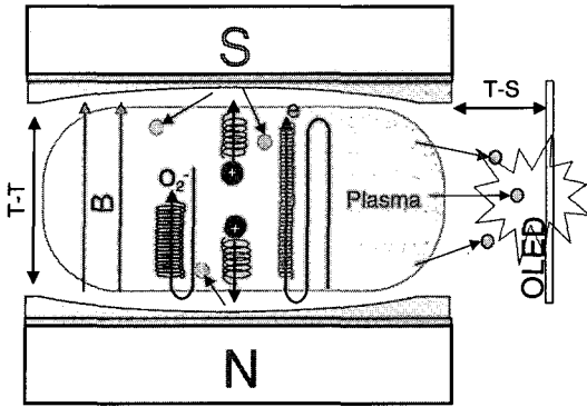
그림 8. 박스 캐소드 스퍼터의 플라즈마 데미지 프리 성막 기구.
