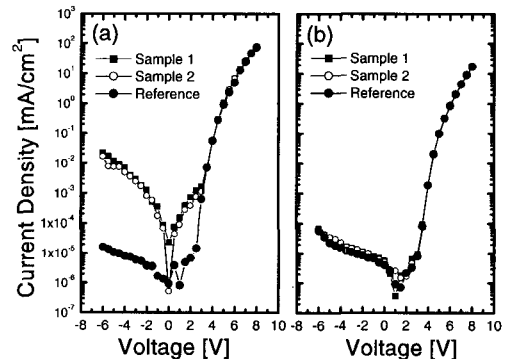
그림 3. (a) DC 마그네트론 스퍼터로 제작된 Al 전극을 가진 OLED와 (b) 박스 캐소드 스퍼터로 제작된 Al전극을 가진 OLED의 전류-전압 특성.
