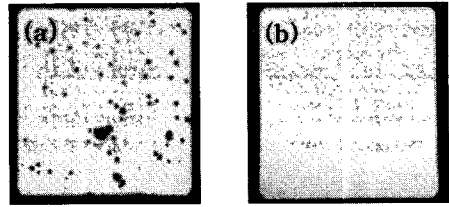
그림 5. (a) DC 마그네트론 스퍼터로 제작된 Al 전극을 가진 OLED와 (b) 박스 캐소드 스퍼터로 제작된 Al전극을 가진 OLED의 EL 이미지. Fig. 5. EL images of OLED prepared by (a) DC magnetron sputtering and (b) box cathode sputtering, respectively.
