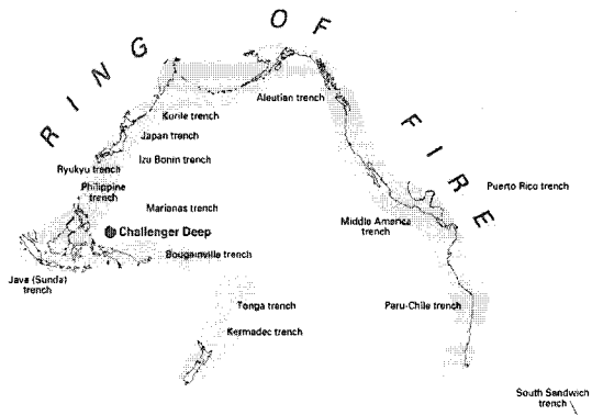
그림 2. 환태평양 지진대 및 알프스-히말라야 지진대
