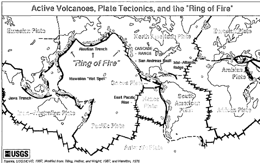
그림 3. 판구조론에 의한 판경계 및 관련 지진 및 화산대
