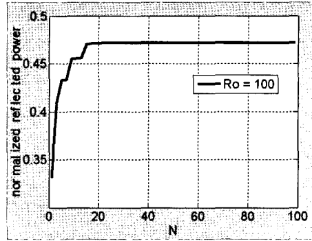
그림 4. 수직입사 시 N에 따른 정규화된 반사전력 수렴곡선 Fig. 4. The convergence curve of the normalized reflected power vs. N for normal incidence
