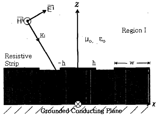
그림 1. 균일한 저항율의 저항띠 격자구조에 임의의 방향으로 입사되는 H-분극 평면파 Fig. 1. H-polarized plane wave with oblique incidence on a resistive strip grating with uniform resistivity
