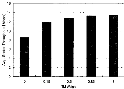
그림 18. Unified Metric을 이용한 OFDM/SDMA 기반 자원 할당 알고리즘의 평균 섹터 Throughput (SCME Urban Macro 1 3km/h, Case II) Fig. 18. The Average Sector Throughput of OFDM/SDMA based Resource Allocation Algorithm utilizing Unified Metric. (SCME Urban Macro 1 3km/h, Case II)
