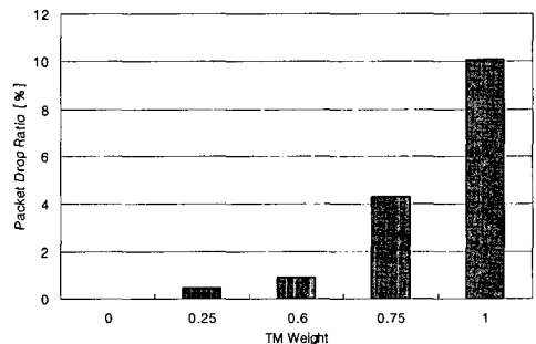
그림 17. Unified Metric을 이용한 OFDM/SDMA 기반 자원 할당 알고리즘을 적용한 경우, 실시간 서비스 사용자의 Packet Drop Ratio (SCME Urban Macro 1 3km/h, Case I) Fig. 17. The Average Packet Drop Ratio of OFDM/SDMA based Resource Allocation Algorithm utilizing Unified Metric. (SCME Urban Macro 1 3km/h, Case I)
