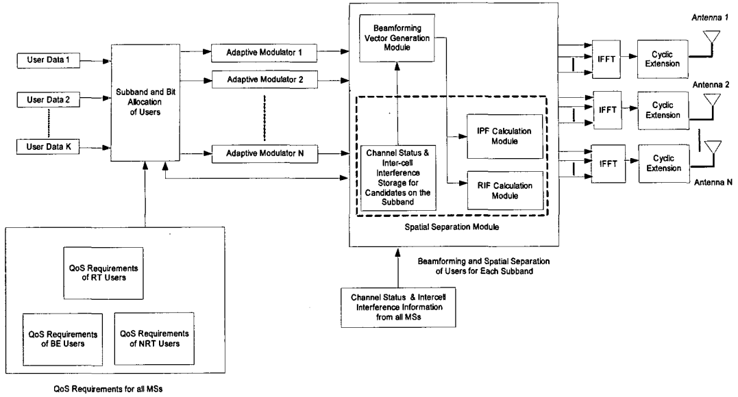
그림 1. 제안하는 OFDM/SDMA 기반 기지국 시스템 블록 다이어그램 Fig. 1. The Block Diagram of the Proposed OFDM/SDMA Transmitter
