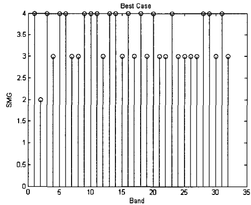
그림 7. SDMA 알고리즘의 Spatial Multiplexing Gain (5 사용자 / 섹터, 평균 SINR = 33dB) Fig. 7. Spatial Multiplexing Gain of SDMA Algorithm (5Users / Sector, Average SINR = 33dB)
