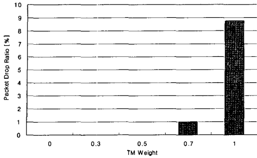
그림 13. Unified Metric을 이용한 OFDM/SDMA 기반 자원 할당 알고리즘을 적용한 경우, 실시간 서비스 사용자의 Packet Drop Ratio. (Ped A 3km/h, Case I) Fig. 13. The Average Packet Drop Ratio of OFDM/SDMA based Resource Allocation Algorithm utilizing Unified Metric. (Ped A 3km/h, Case I)
