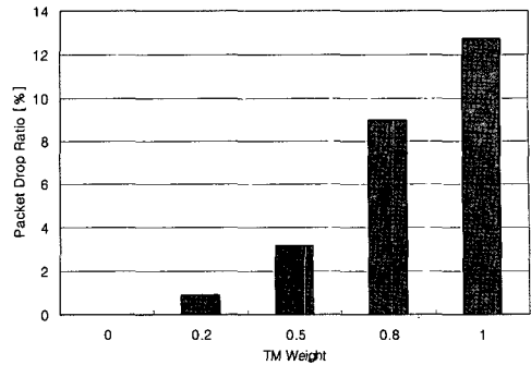
그림 15. Unified Metric을 이용한 OFDM/SDMA 기반 자원 할당 알고리즘을 적용한 경우, 실시간 서비스 사용자의 Packet Drop Ratio. (Ped A 3km/h, Case II) Fig. 15. The Average Packet Drop Ratio of OFDM/SDMA based Resource Allocation Algorithm utilizing Unified Metric. (Ped A 3km/h, Case II)
