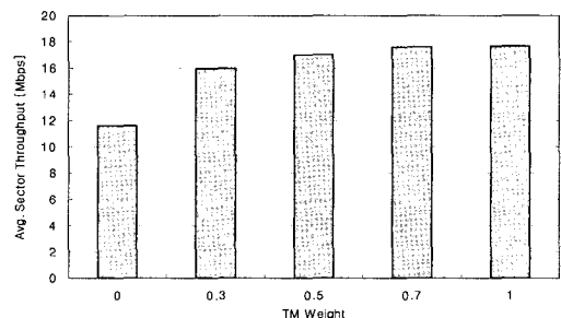
그림 12. Unified Metric을 이용한 OFDM/SDMA 기반 자원할당 알고리즘의 평균 섹터 Throughput. (Ped A 3km/h, Case I) Fig. 12. The Average Sector Throughput of OFDM/SDMA based Resource Allocation Algorithm utilizing Unified Metric. (Ped A 3km/h, Case I)
