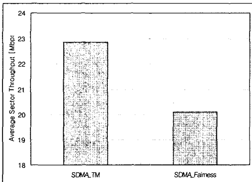
그림 9. Throughput 최대화 기반 SDMA 알고리즘과 Fairness 기반 SDMA 알고리즘 적용 시 섹터 Throughput 비교 Fig. 9. Comparison of Sector Throughput between SDMA Algorithm based on Throughput Maximization and SDMA Algorithm based on Fairness
