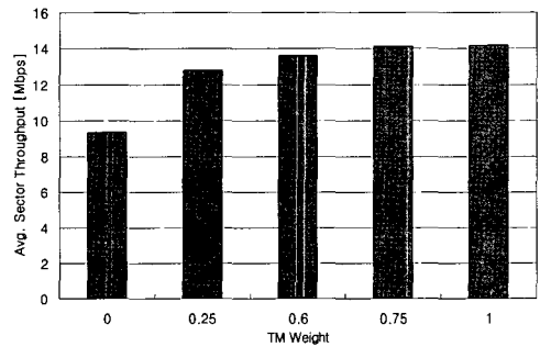
그림 16. Unified Metric을 이용한 OFDM/SDMA 기반 자원 할당 알고리즘의 평균 섹터 Throughput (SCME Urban Macro 1 3km/h, Case I) Fig. 16. The Average Sector Throughput of OFDM/SDMA based Resource Allocation Algorithm utilizing Unified Metric. (SCME Urban Macro 1 3km/h, Case I)
