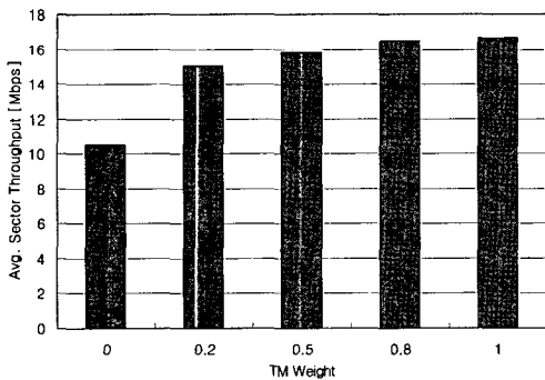
그림 14. Unified Metric을 이용한 OFDM/SDMA 기반 자원 할당 알고리즘의 평균 섹터 Throughput. (Ped A 3km/h, Case II) Fig. 14. The Average Sector Throughput of OFDM/SDMA based Resource Allocation Algorithm utilizing Unified Metric. (Ped A 3km/h, Case II)
