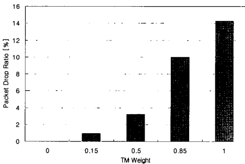
그림 19. Unified Metric을 이용한 OFDM/SDMA 기반 자원 할당 알고리즘을 적용한 경우, 실시간 서비스 사용자의 Packet Drop Ratio (SCME Urban Macro 1 3km/h, Case II). Fig. 19. The Average Packet Drop Ratio of OFDM/SDMA based Resource Allocation Algorithm utilizing Unified Metric. (SCME Urban Macro 1 3km/h, Case II)
