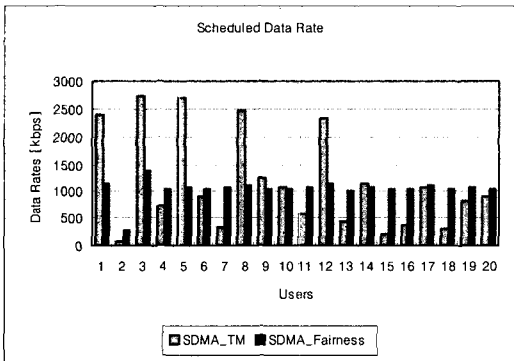
그림 8. 각 사용자별 자원 할당 분포 Fig. 8. Scheduled Data Rate per User
