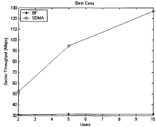
그림 6. DL Sector Throughput 비교 (평균 SINR = 33dB) Fig. 6. Comparison of DL Sector Throughput (Average SINR = 33dB)
