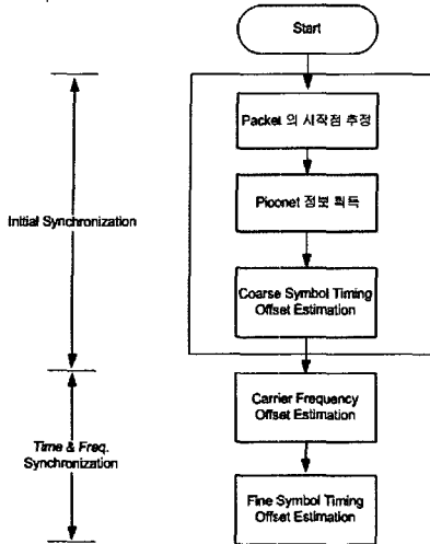
그림 3. UWB MB-OFDM 시스템 동기화 과정
