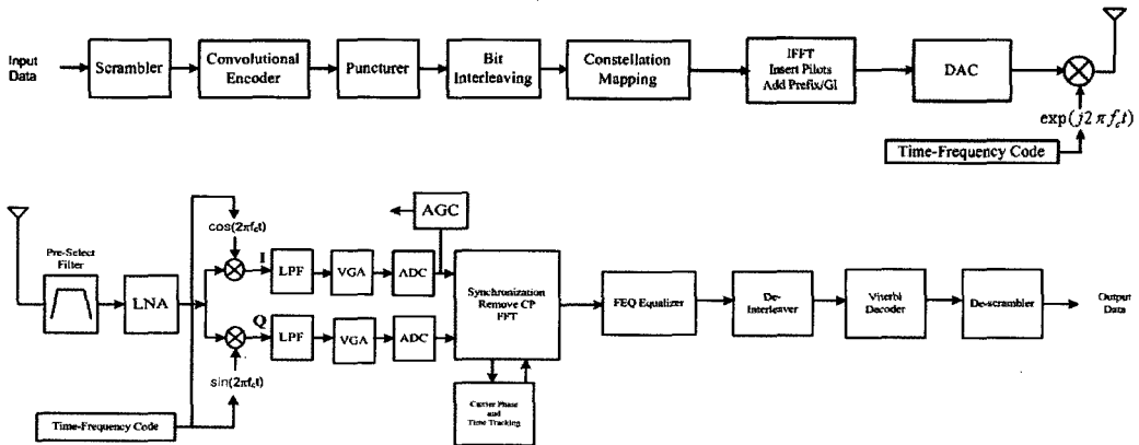
그림 1. UWB MB-OFDM 모델의 구조
