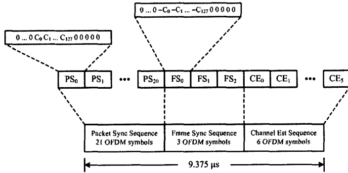
그림 2. UWB MB-OFDM 프리앰블 구조
