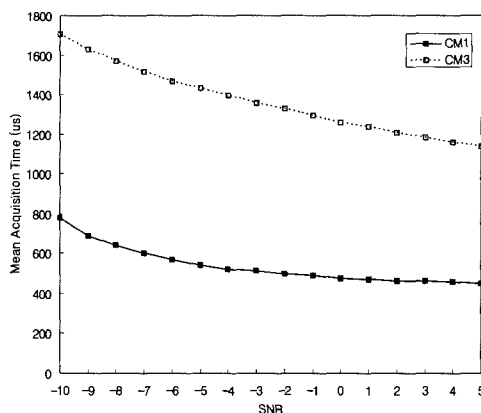
그림 5. CM 1 및 CM 3 환경에서의 Packet Detection 및 Piconet 정보 추정 성능
