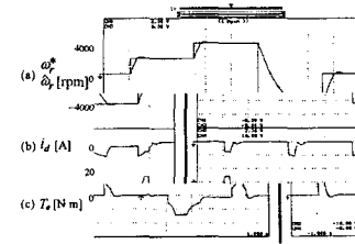
그림 15 스텝 지령속도에 변화에 대한 FNN의 응답특성 Fig. 15 Response characteristics of FNN in command speed change
