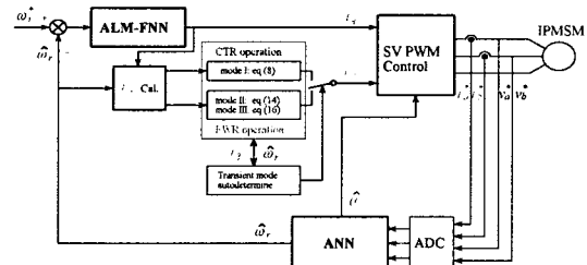
그림 6 AI 제어기에 의한 최대토크 제어기의 전체 블록도 Fig. 6 The block diagram of maximum torque controller with AI controller
