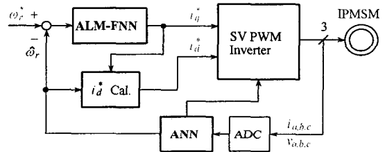
그림 3 CTR에서 드라이브 시스템의 제어 블록도 Fig. 3 Control block diagram of drive system in CTR
