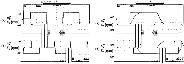
그림 19 스텝 지령속도 변화에 최대토크 제어 응답 특성
