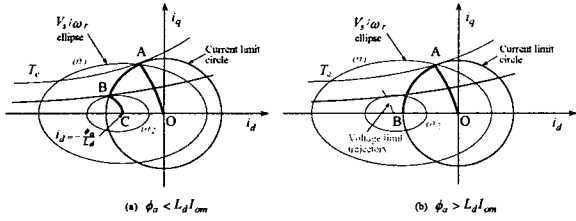
그림 4 전동기의 동작 모드 Fig. 4 Operating mode of motor
