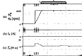
그림 7 스텝 지령속도에 대한 I_d=0 제어의 응답특성 Fig. 7 Response characteristics of I_d=0 with step command speed
