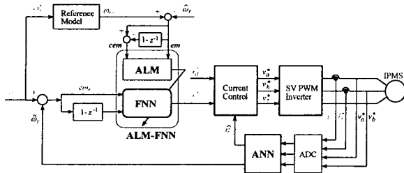
그림 5 AI 제어기 Fig. 5 AI controller
