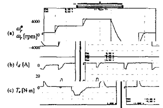
그림 16 스텝 지령속도에 변화에 대한 ALM-FNN의 응답특성 Fig. 16 Response characteristics of ALM-FNN in command speed change
