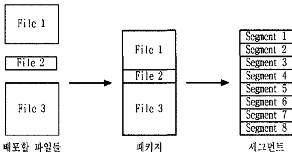
(그림 1) 배포할 파일들, 패키지, 세그먼트의 관계
