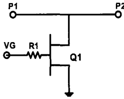
(a) FET 스위치 설계를 위한 4F200 pHEMT의 병렬 구조 (a) Shunt structure of 4F200 pHEMT to design FET switch
