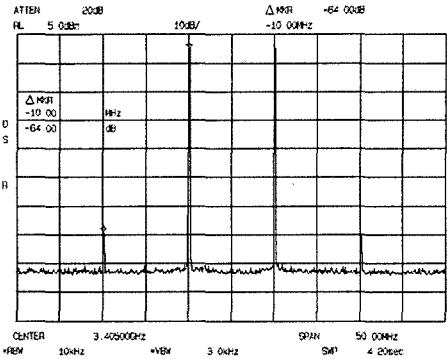
그림 8. 제작된 스위치 MMIC의 IMD3 측정 결과 Fig. 8. Measured IMD3 Result of the fabricated MMIC
