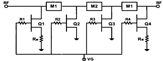
그림 2. 새로운 흡수형 SPST FET 스위치 구조 Fig. 2. Proposed configuration of absorptive SPST FET switch
