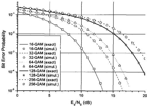
그림 4. QAM의 각 변조 차수에 따른 성능 비교: 연관정 결과와 QAM 성능 계산식을 이용한 계산한 결과 비교
