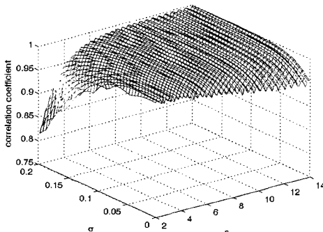
그림 3. 매질투과시 변형된 신호와 원래신호간의 상관계수. 매질의 두께는 20cm로 가정하였다.
