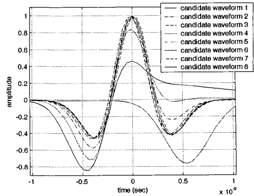
그림 6. LBG 알고리즘을 이용하여 얻어진 대표 파형( N=8 ). 신호의 energy는 정상화되어 있다.
