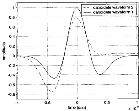
그림 4 LBG 알고리즘을 이용하여 얻어진 대표 파형( N=2 ). 신호의 energy는 정상화되어 있다.
