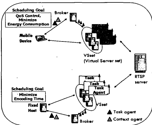
그림 1. 유비쿼터스 멀티미디어 서비스 환경
