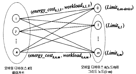
그림 4. 소프트웨어 재구성의 플로우 네트워크
