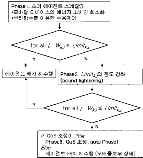
그림 5. RtoA의 소프트웨어 재구성 다이어그램
