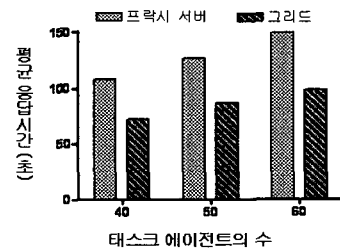
그림 15. 에이전트의 평균 응답시간
