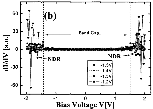
그림 4 Nitro-benzenethiolate의 (a) I-V 특성 (b) dI/dV 특성 Fig. 4 Characteristic of (a) I-V and (b) dI/dV of nitro-benzenethiolate
