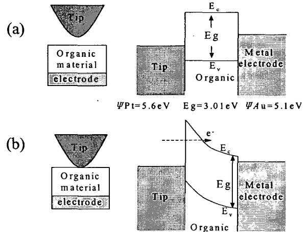
그림 5 STM tunneling에 의한 에너지 다이어그램 (a) 전압을 인가하기 전 평형상태 (b) 전압을 인가했을때 다이어그램 Fig. 5 Energy diagrams for STM tunneling (a) before bias voltage and (b) after bias voltage
