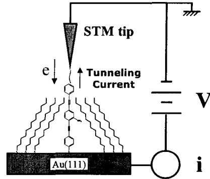
그림 2 STM 및 STS 측정시스템 모식도 Fig. 2 Schematic diagram of STM and STS measurement system
