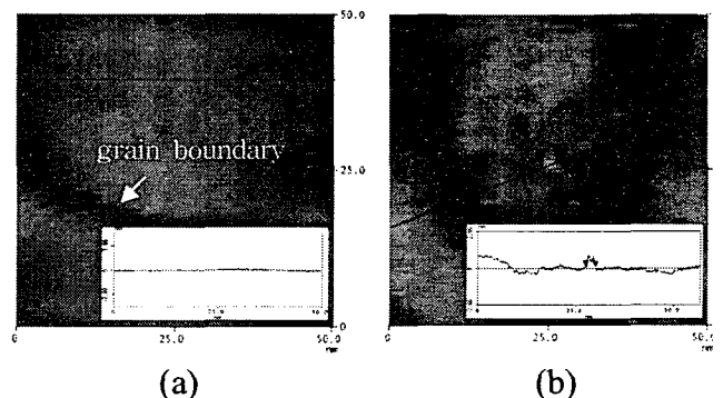
그림 3 STM 이미지 (a) bare 상태의 Au (111) 이미지 (b) SAMs의 표면 이미지 Fig. 3 STM images of (a) bare Au(111) substrate and (b) self-assembled organic monolayer
