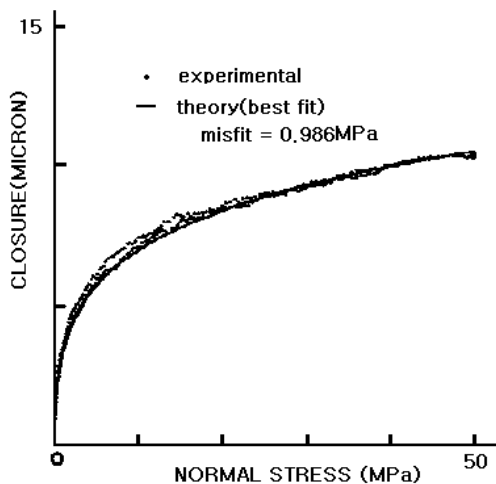
Fig. 3 응력에 따른 두 석재 간 간격의 변화.
