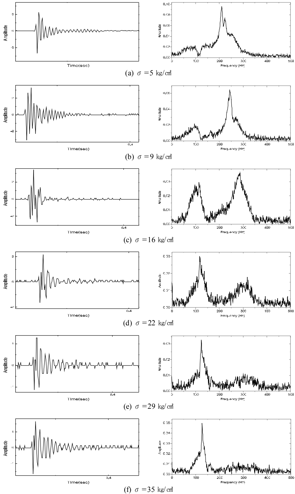
Fig. 8 축하중 증가에 따른 석벽돌 적층모델의 1차 고유진동수 변화.
