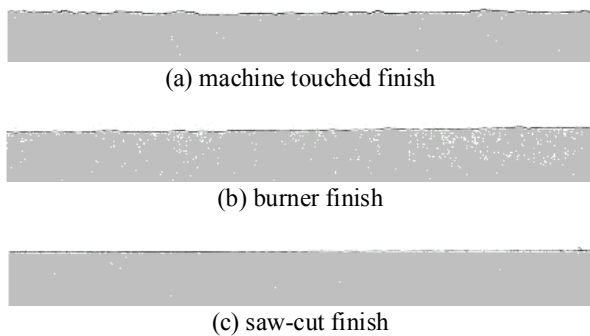
Fig. 6. 석벽돌 표면의 Profile.
