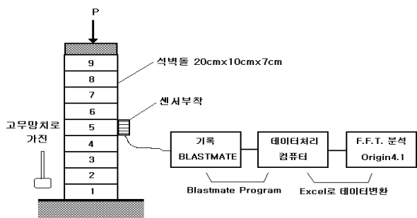
Fig. 7 실험 개념도.
