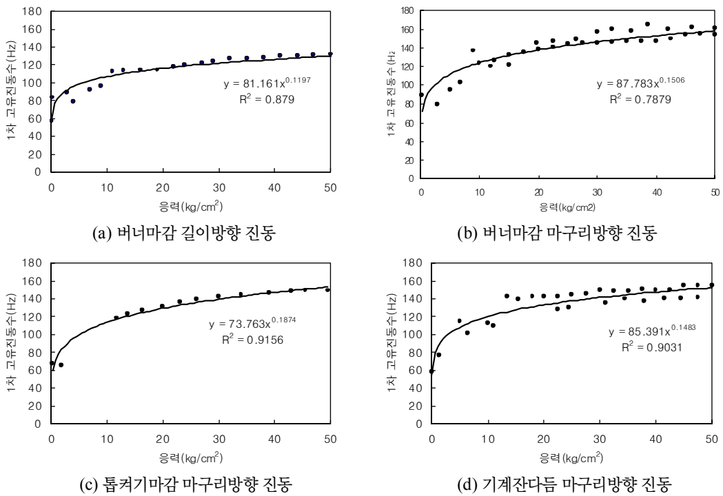
Fig. 10 석벽돌 적층모델의 마감과 진동방향에 따른 1차 고유진동수.
