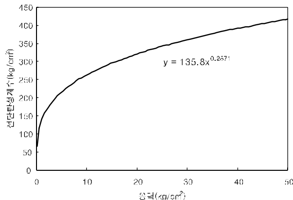
Fig. 13 끼움 기둥 부재의 축응력에 따른 전단탄성계수.
