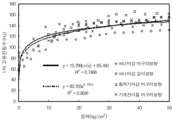
Fig. 9 축응력-1차 고유진동수 측정결과(종합).
