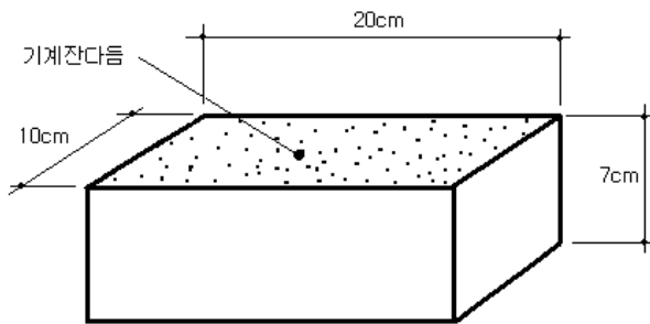
Fig. 5 석벽돌 시료의 제원.
