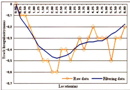
그림 4. Application example of Smoothing Filter
