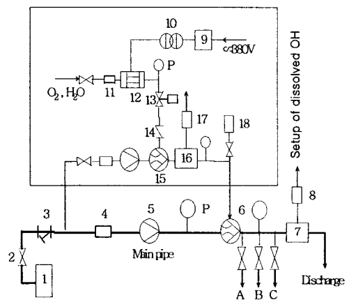
(1) 선박안정수용기, (2) 인입밸브(O 2 +H 2 O), (3) 필터, (4) 유량계, (5) 펌프, (6) 용액/용액 용해기, (7)및(16) 가스/용액 분리기, (8)및(17) 용존 OH 여과기, (9) 제어기, (10) 변압기, (11) 유량계, (12) OH 플라즈마 반응기, (13) 자동밸브, (14) 검사밸브, (15) 가스/용액 용해기, (18) OH 검출기
