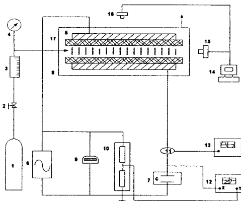
(1) 가스통, (2) 레귤레이터, (3) 유량계, (4) 압력계, (5) DBD 장치, (6) 교류전원, (7) 정전용량, (8) 차폐용기, (9) 정전원장치, (10) 압력계, (11) 전류계, (12) X-Y 레코더, (13) 오실로스코프, (14) 컴퓨터, (15), (16) CCD, (17) 출기구, (18) 배기구
