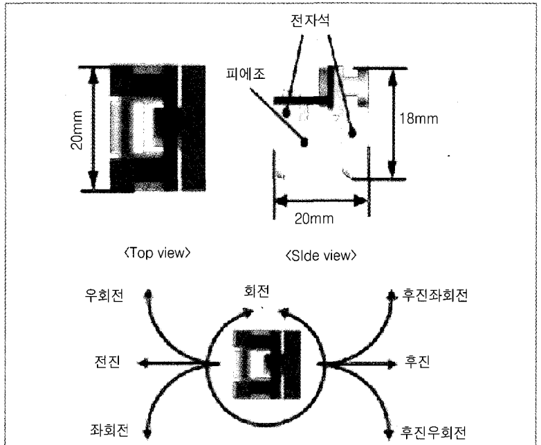
그림 8 마이크로 로봇의 구동원리
