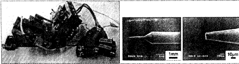
그림 5 마이크로 포밍 시스템
