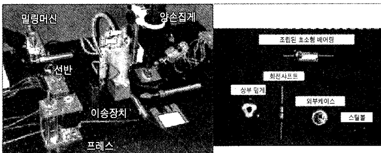
그림 2 초소형 부품용 마이크로 팩토리
