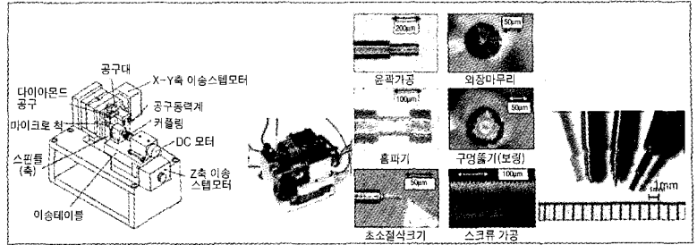
그림 3 일본에서 제작된 마이크로 선반
