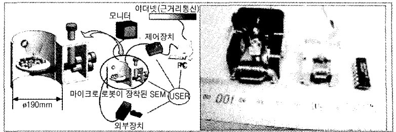
그림 7 SEM 진공챔버 안에서의 마이크로 시스템
