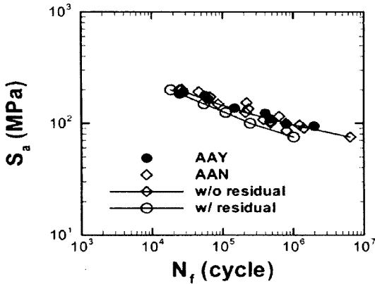
Fig. 9 Butt weld
