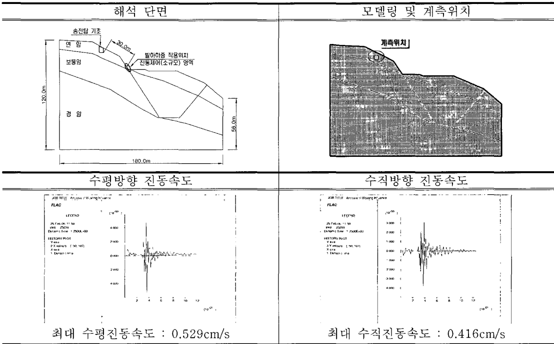
그림 5. 진동제어(소규모) 발파시 해석결과.
