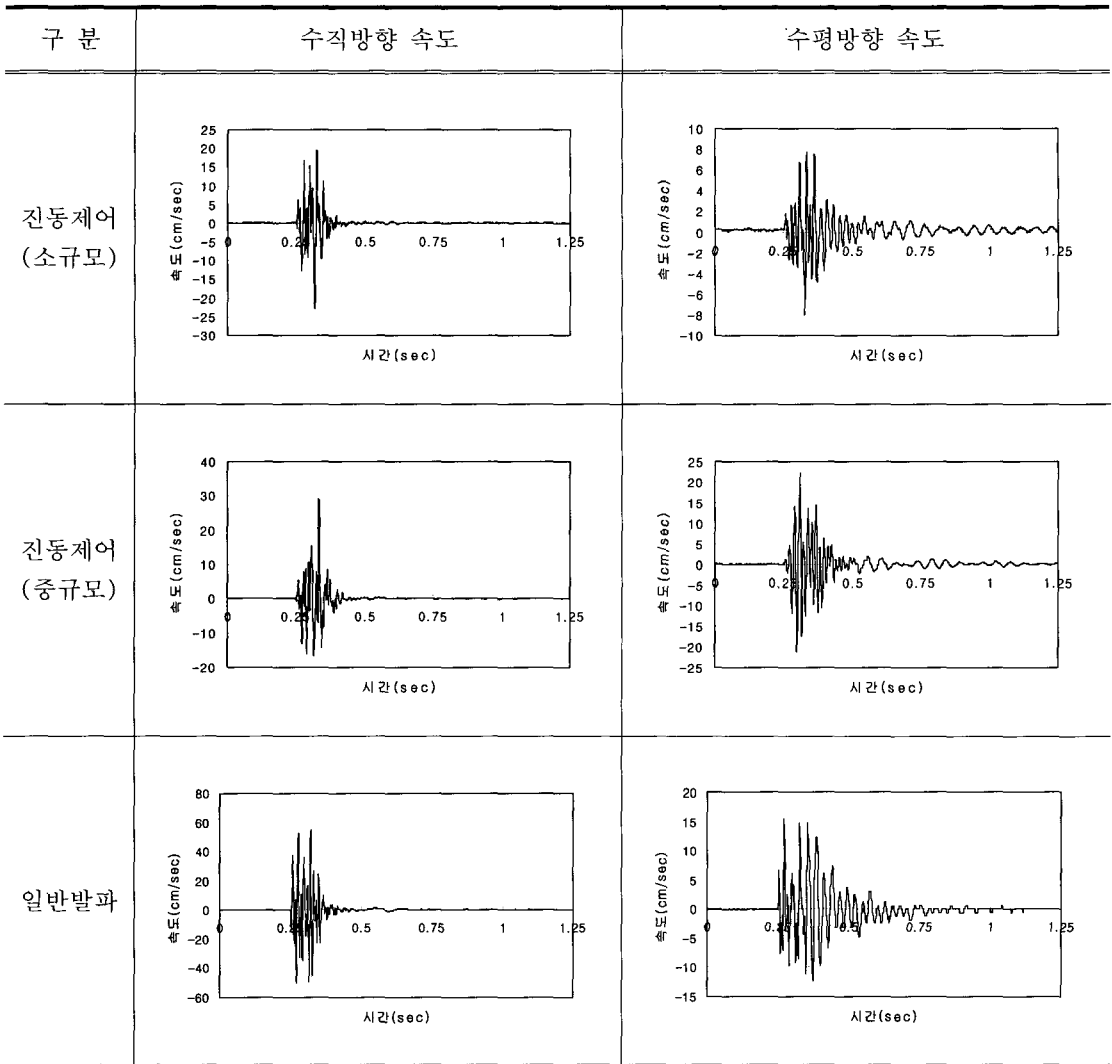
그림 4. 각 발파공법별 보정된 수치해석 적용 진동과형.
