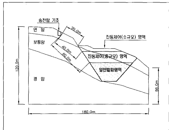
그림 2. 발파진동 해석단면 및 적용 발파패턴.
