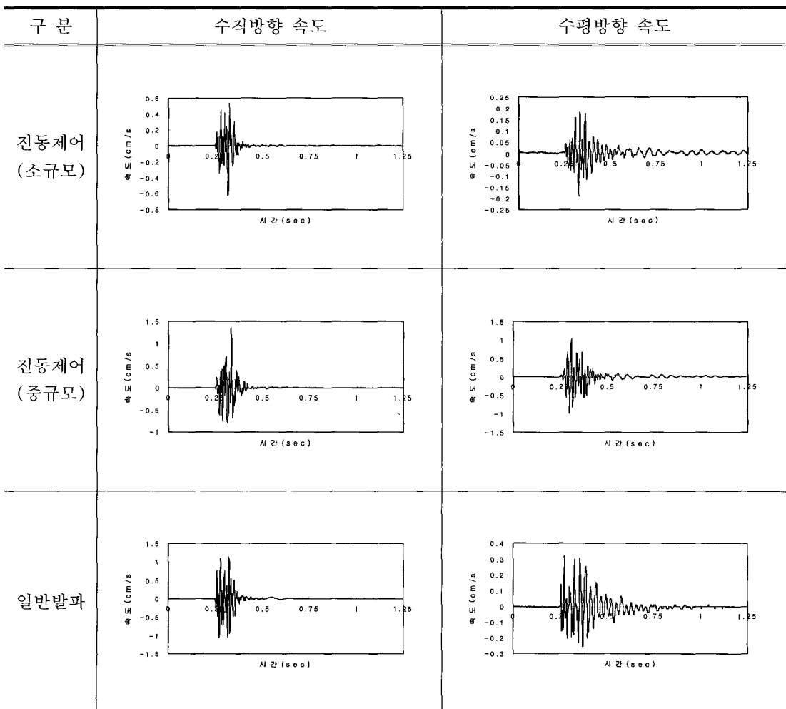
그림 3. 각 발파공법별 적용한 실측진동파형.
