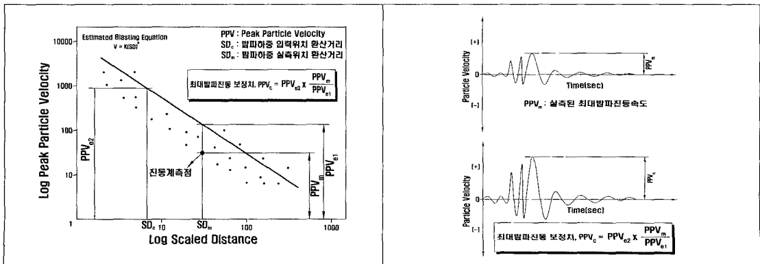
그림 1. 시험발파시 측정된 진동파형을 이용한 발파하중 산정방법.
