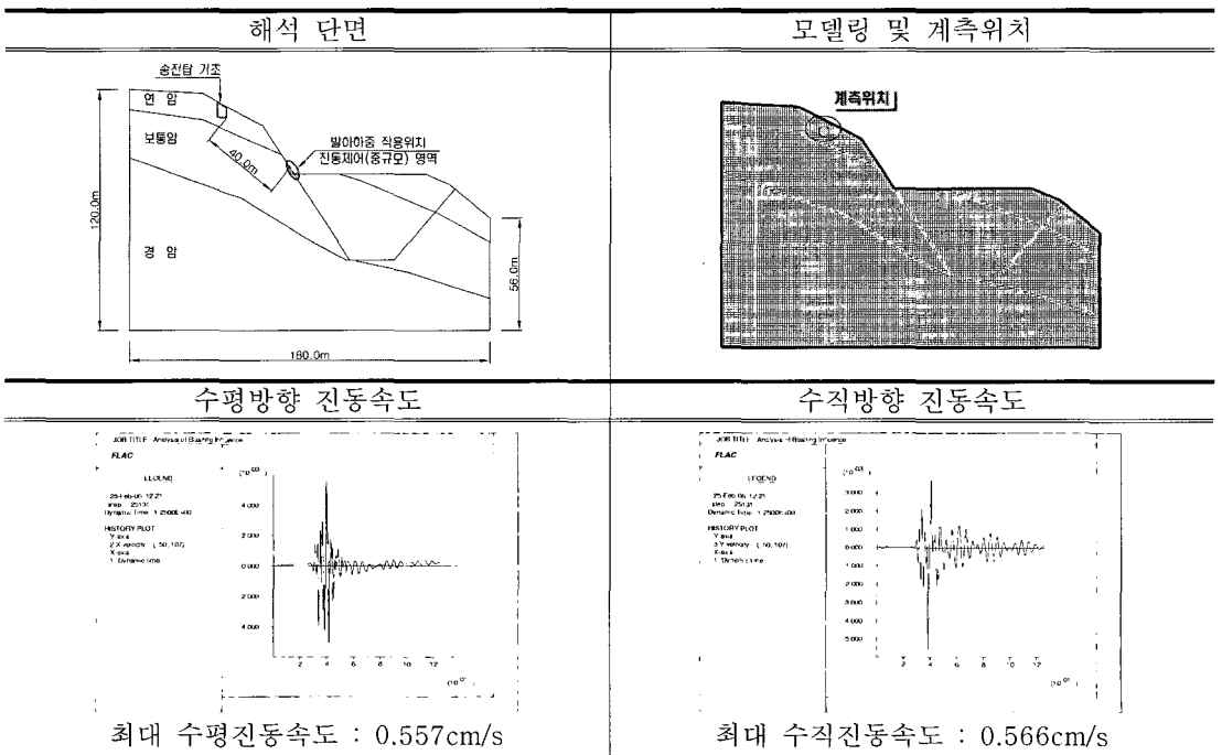
그림 6. 진동제어(중규모) 발파시 해석결과.
