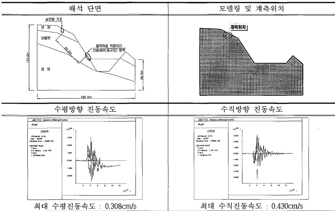
그림 7. 일반 발파시 해석결과.
