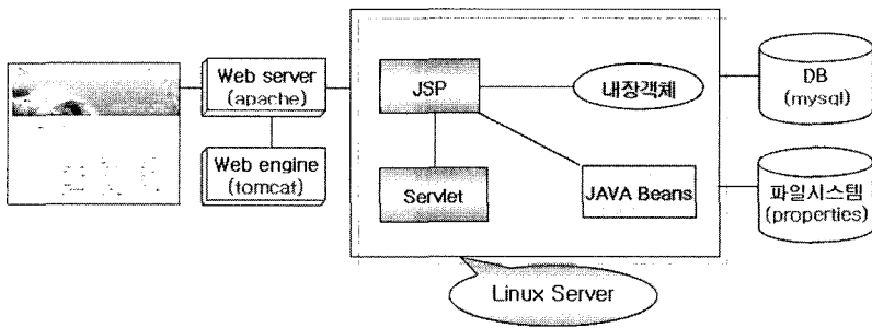
〈그림 21〉 시스템 구성도
