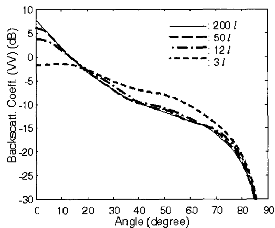
그림 11. 표면 길이에 따른 VV-편파의 후방 산란 계수 비교( k_s=1 , k_l=10 )
