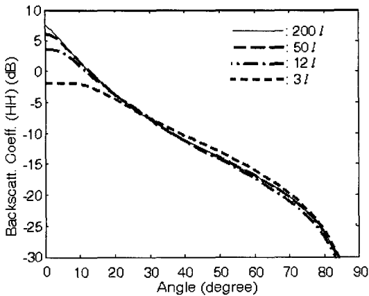
그림 10. 표면 길이에 따른 HH-편파의 후방 산란 계수 비교( k_s=1 , k_l=10 )
