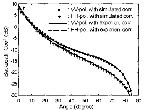
그림 9. 이론적, 수치 해석적 후방 산란 계수들의 비교( ks=1 , kt=10 ) Fig. 9. Comparison between analytical and numerical backscattering coefficients.
