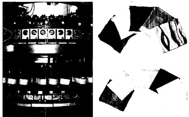
그림 6. 전자식 자카드 선침기구인 WAC과 환편 자카드 직물
