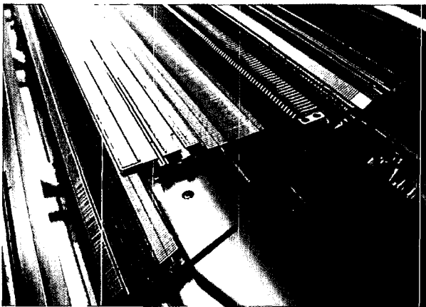
그림 2. Shima Seiki사 무봉제기의 X-type 4단 베드
