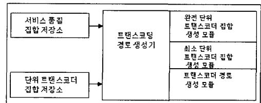
그림 2. 단위 트랜스코더 집합을 고려한 응용 독립적 멀티미디어 적응 프레임워크의 모델
