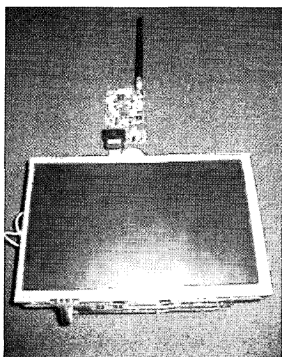
그림 6 베이스노드와 게이트웨이 연결 fig 6. Base node and gateway connection
