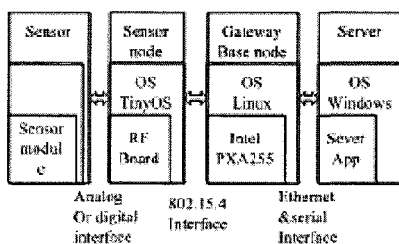
그림 7. 소프트웨어 모듈 구조 fig 7. Software module structure
