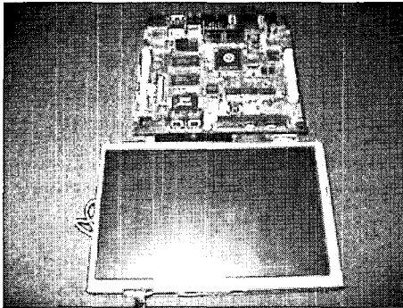
그림 8 게이트웨이(임베디드 리눅스 탑재) Fig 8. Gateway(Embedded linux installed)
