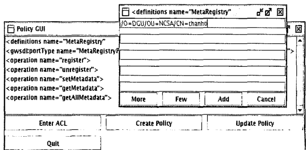
(그림 12) 접근 제어 리스트에 항목 추가
