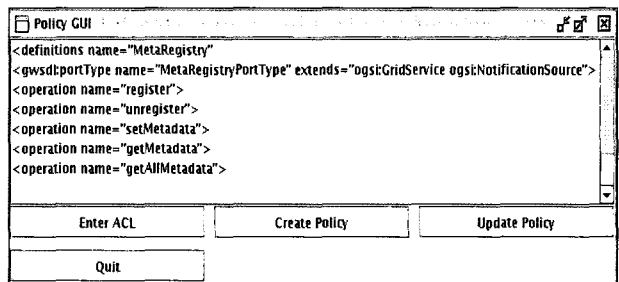
(그림 11) 정책관리자 툴
