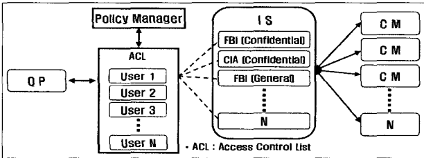
(그림 10) 제한된 시스템의 구조
