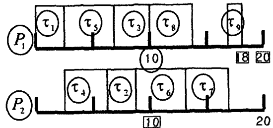
그림 5 프로세스 P2의 태스크 스케줄
