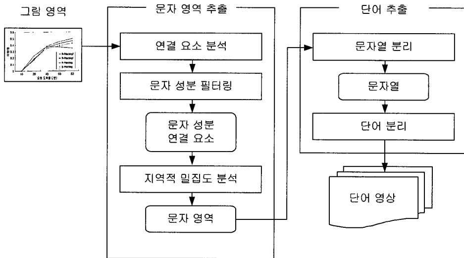
(그림 3.1) 그림 영역에서 단어 영상 추출의 단계별 수행 과정
