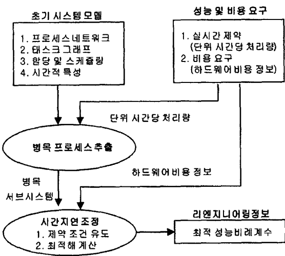
그림 1 시스템 리엔지니어링 과정
