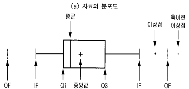
(a) 자료의 분포도
