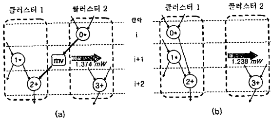
그림 3 연산 할당의 효과를 보여주는 예제
