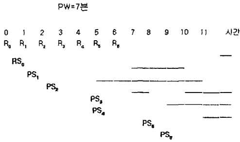
(a) R_0 \sim R_6 요청의 서비스 시작시간과 패킹 스트림
