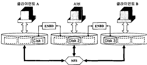
(그림 5) 프리웨어를 이용한 SIOS
