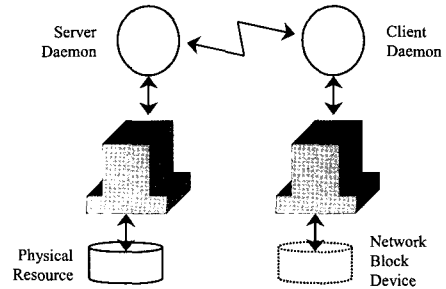
(그림 4) NBD를 이용한 원격 디스크 접근
