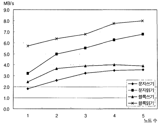
(그림 8) 다중 노드 액세스에 따른 I/O 처리율
