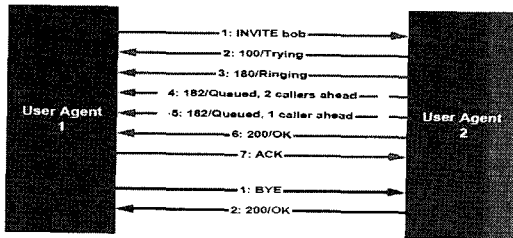
그림 2. SIP INVITE 메시지 요청과 응답 Fig. 2 SIP INVITE Message Request and Response
