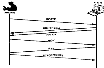
그림 6. 콜 스팸 연결 Fig. 6 Call Spam Connect
