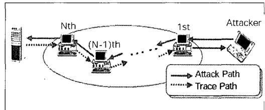
그림 9 VoIP 네트워크 보안 시스템에서의 역추적 차단 Fig. 9 Cut off Traceback at VoIP Network Security Systems
