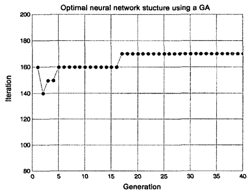
Fig. 6 Optimal iteration
