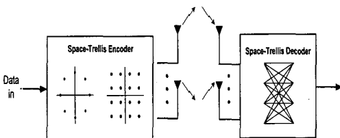
그림 2. SFTC-OFDM 방식의 블록도
