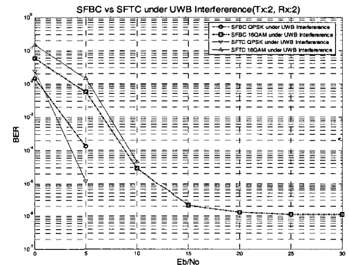
(b) MB-OFDM UWB Interferer가 있는 환경에서의 SFBC-OFDM(Tx:2, Rx:2)와 SFTC-OFDM(Tx:2, Rx:2) 성능
