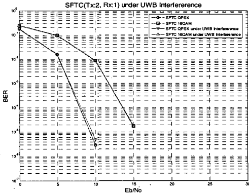
(a) MB-OFDM UWB Interferer가 있는 환경에서의 SFTC-OFDM(Tx:2, Rx:1) 성능 비교
