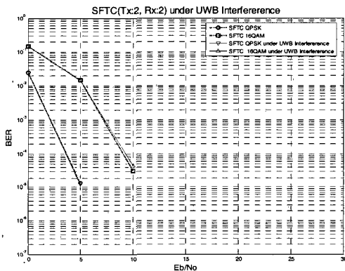
(b) MB-OFDM UWB Interferer가 있는 환경에서의 SFTC-OFDM(Tx:2, Rx:2) 성능 비교
