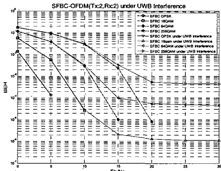
(b) MB-OFDM UWB Interferer가 있는 환경에서의 SFBC-OFDM(Tx:2, Rx:2) 성능
