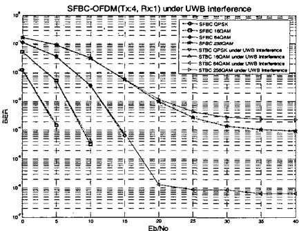
(c) MB-OFDM UWB Interferer가 있는 환경에서의 SFBC-OFDM(Tx:4, Rx:1) 성능
