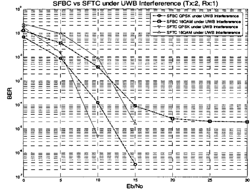
(a) MB-OFDM UWB Interferer가 있는 환경에서의 SFBC-OFDM(Tx:2, Rx:1)와 SFTC-OFDM(Tx:2, Rx:1) 성능
