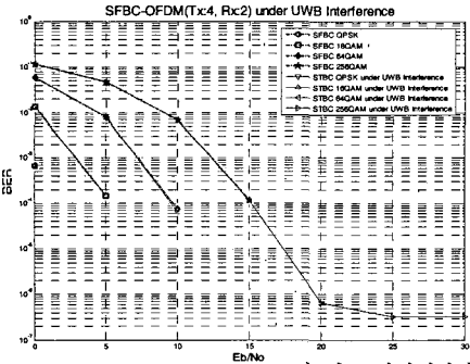
(d) MB-OFDM UWB Interferer가 있는 환경에서의 SFBC-OFDM(Tx:4, Rx:2) 성능
