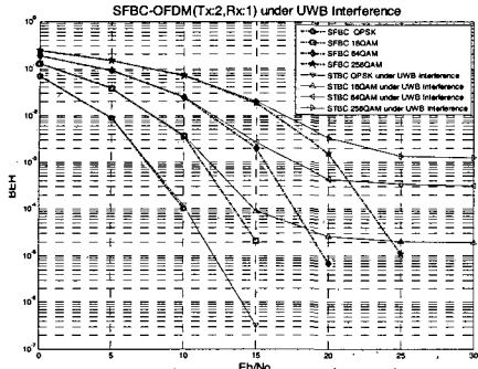
(a) MB-OFDM UWB Interferer가 있는 환경에서의 SFBC-OFDM(Tx:2, Rx:1) 성능
