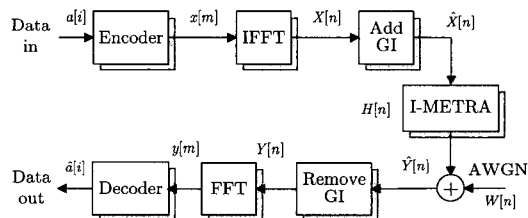
그림 3. OFDM 시스템 구조
