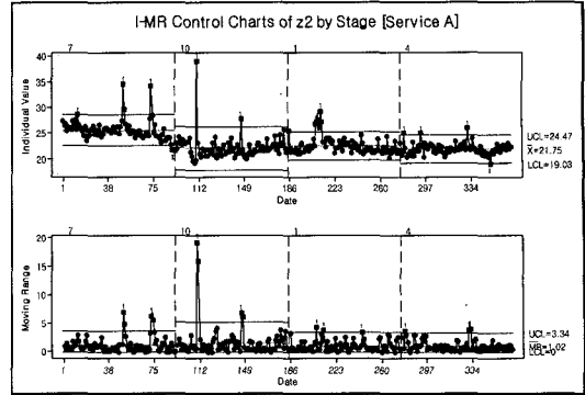
그림 1. I-MR 관리도
