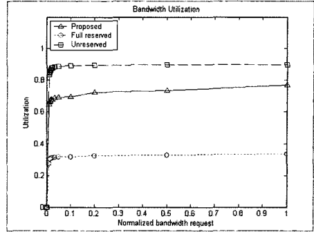
그림 10. Bandwidth Utilization
