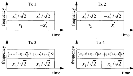
그림 3 C_{3/4} 가진 STF-OFDM의 코딩방식 Fig. 3. Coding scheme of STF-OFDM with C_{3/4}
