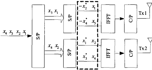
그림 1. 2개의 안테나를 가진 ST-OFDM 송신기의 블록 다이어그램 Fig. 1. Block diagram of two-branch ST-OFDM transmitter
