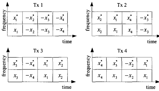
그림 4. 1/2전송율( C_{1/2} )을 가진 STF-OFDM의 코딩방식(T4F2) Fig. 4. Coding scheme of STF-OFDM with C_{1/2} (T4F2)
